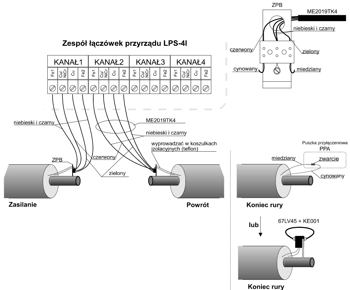
Rysunek poglądowy przedstawiający sposób połączenia miernika LPS-4i za pomocą łączników ZPB z układem alarmowym sieci ciepłej.
