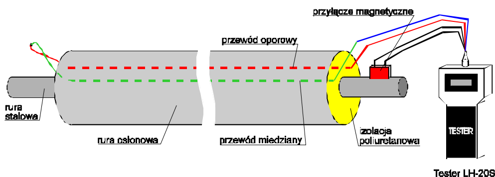
Rys. 1. Pomiar podstawowy.
